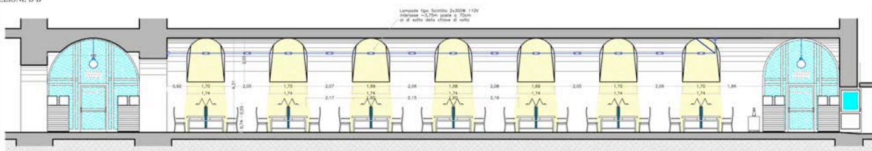
SEZIONE B-B
